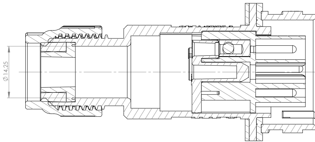
SEZIONE A-A SCALA 2 : 1
