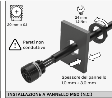
INSTALLAZIONE A PANNELLO M20 (N.C.)
