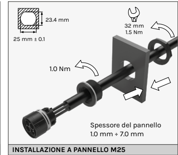
INSTALLAZIONE A PANNELLO M25
